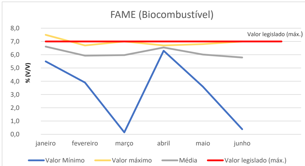
Gráfico 6 - FAME (biocombustível)- Valores máximos mínimos e médios obtidos
