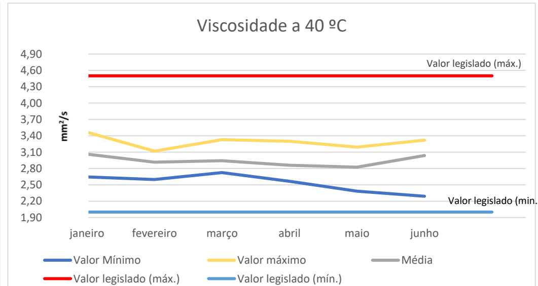
Gráfico 8 - Viscosidade a 40 °C- Valores máximos mínimos e médios obtidos
