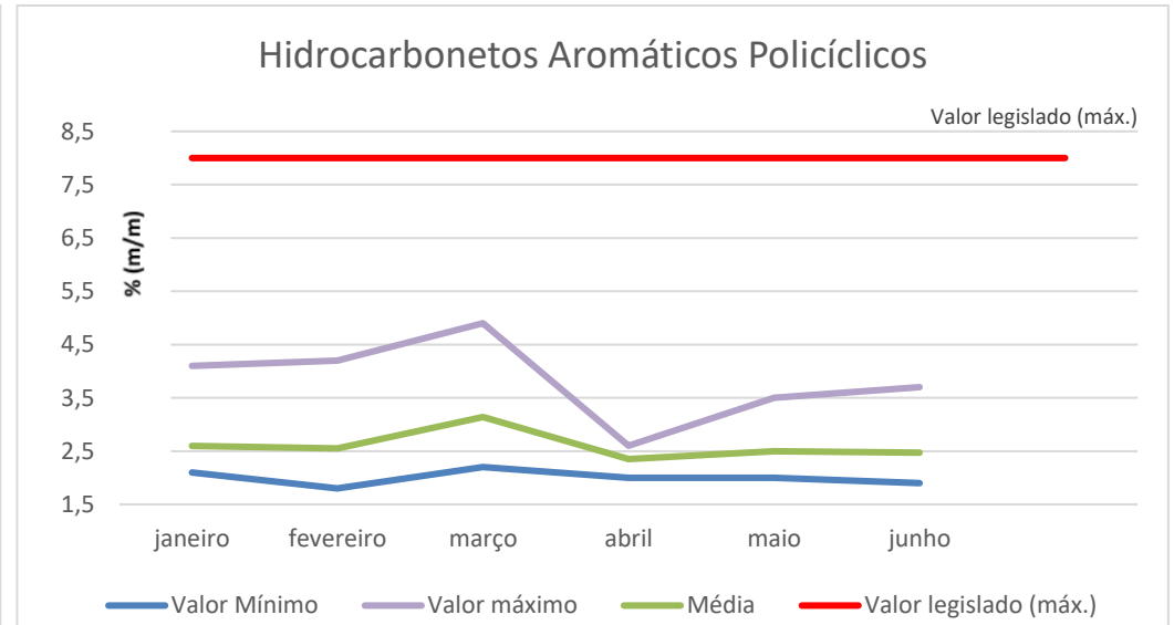
Gráfico 3 - Hidrocarbonetos Aromáticos Policíclicos - Valores máximos mínimos e médios obtidos
