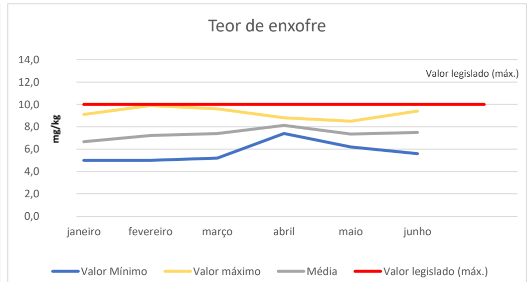
Gráfico 4 - Teor de enxofre - Valores máximos mínimos e médios obtidos
