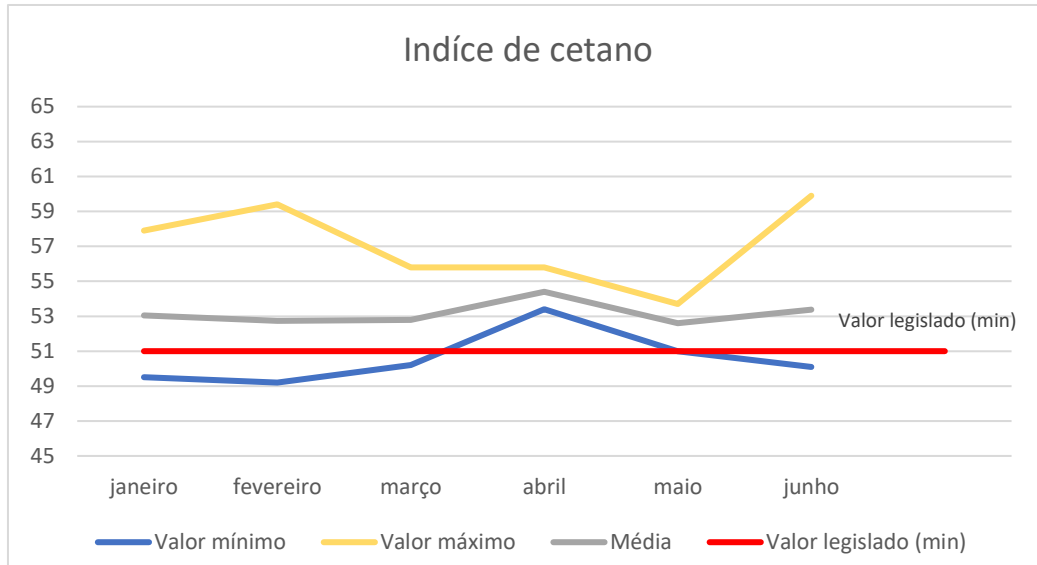
Gráfico 1 - Índice de cetano - Valores máximos mínimos e médios obtidos
