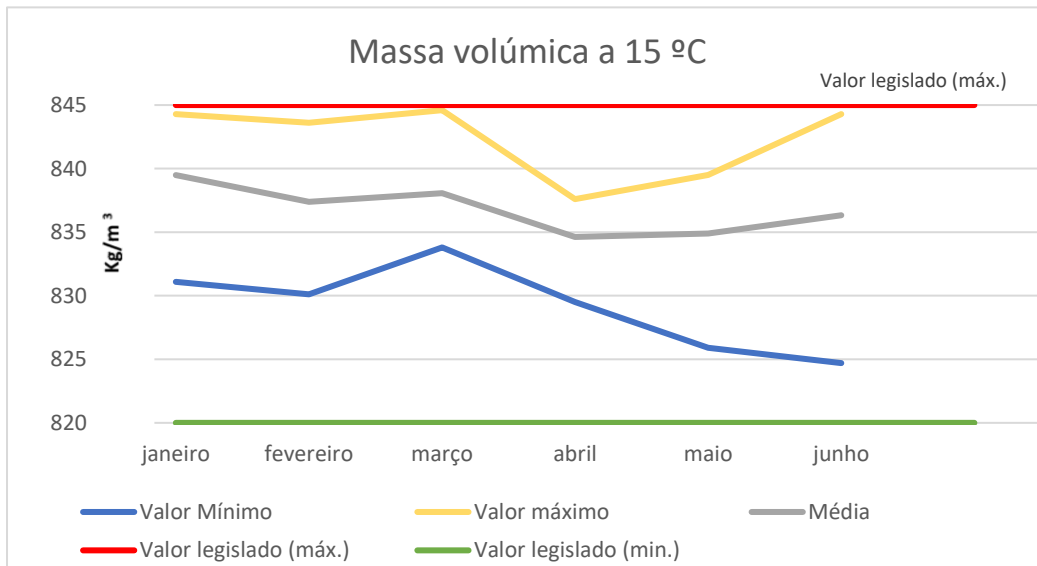
Gráfico 2- Massa volúmica a 15 °C - Valores máximos mínimos e médios obtidos
