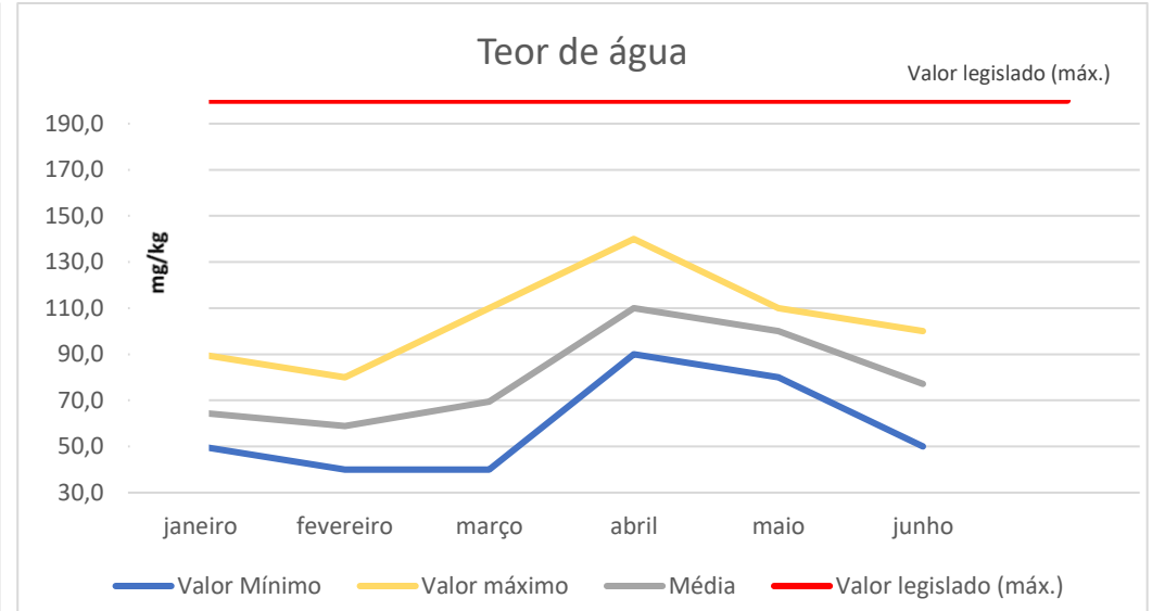
Gráfico 7 - Teor de água- Valores máximos mínimos e médios obtidos
