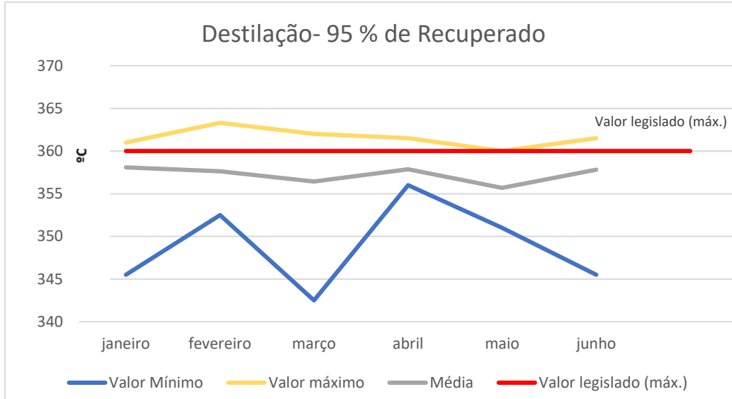
Gráfico 5 - Destilação a 95 % de recuperado- Valores máximos mínimos e médios obtidos
